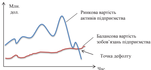
Рис. 2. Ілюстрація основних параметрів моделі Moody's KMV
