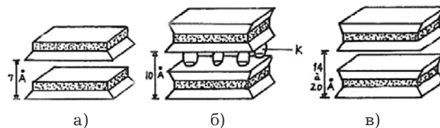
Рис. 1. Структура глинистых минералов: а) каолинита; б) иллита; в) монтмориллонита
