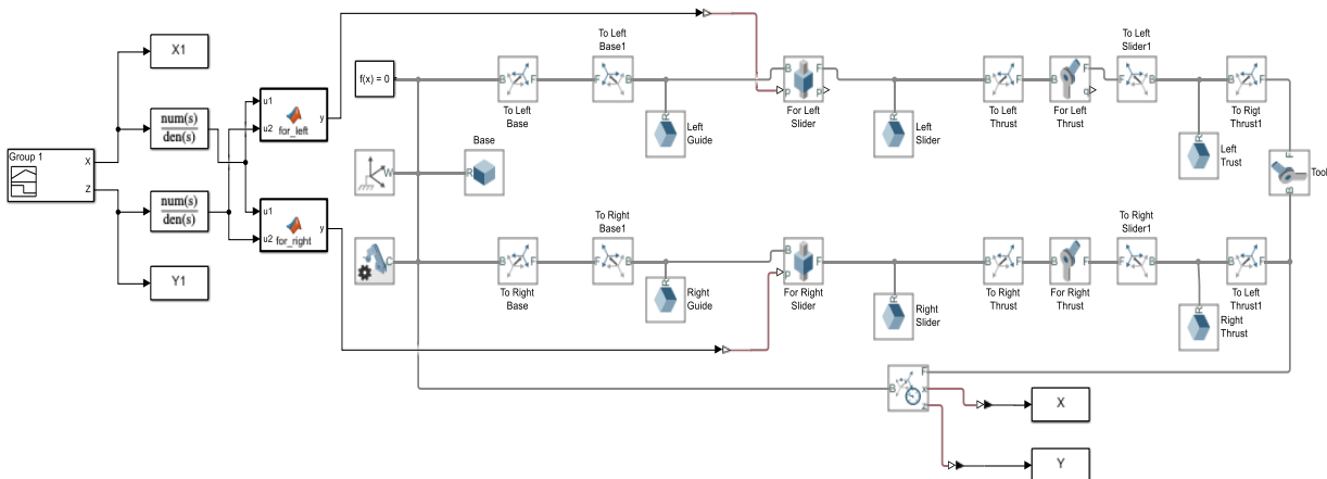
Рис. 2 Математична модель в Simscape Multibody
