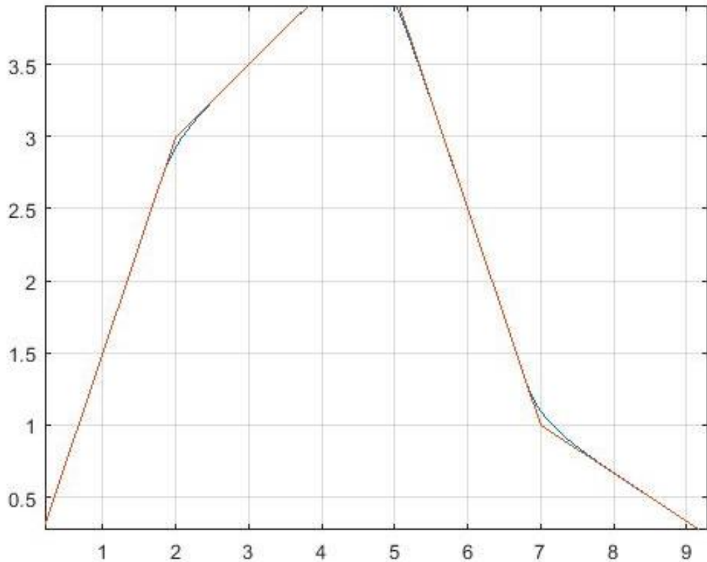
Рис. 3. Результат моделювання відпрацювання принтером заданої траєкторії переміщення робочого органу
