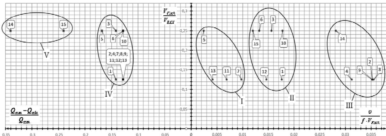
Рис. 1. Двоквадрантна образно-знакова модель визначення ефективного маршрутизатора в безрозмірних координатах Примітка: цифри – 1, 2, ... 13 відповідають порядковому номеру бездротових маршрутизаторів, наведених в табл. 1.
