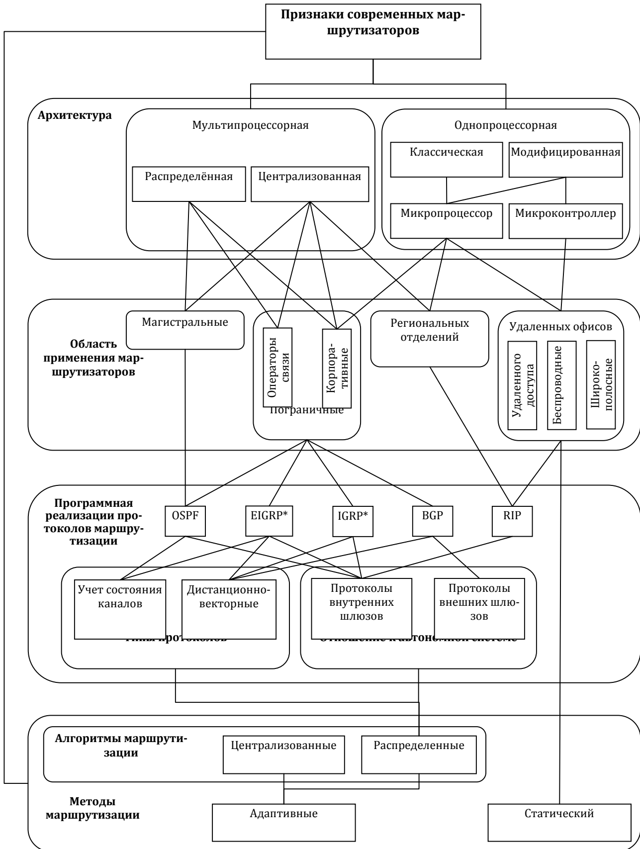
Рис. 3 . Класифікаційна схема сучасних маршрутизаторов
