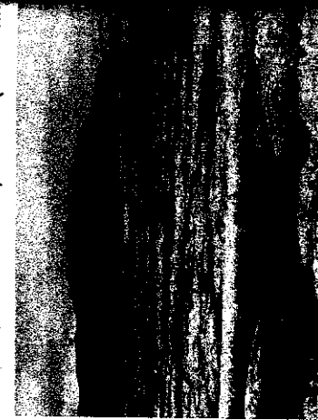
Поднятия морского дна во время Невельского землетрясения (Сахалин)
