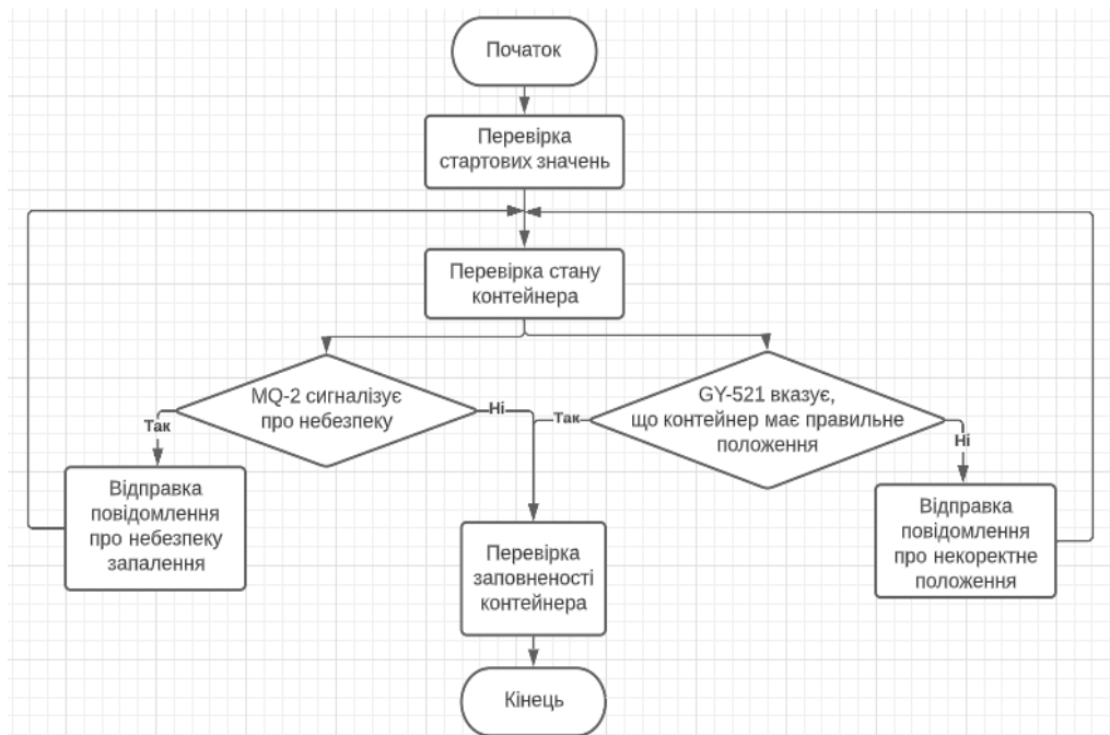
Рисунок 1 – Блок-схема роботи програмного забезпечення системи IoT рішення
