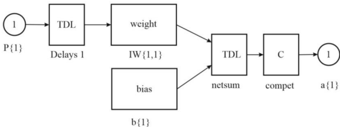
Рисунок 2 – Функції і архітектура мережі Кохонена
