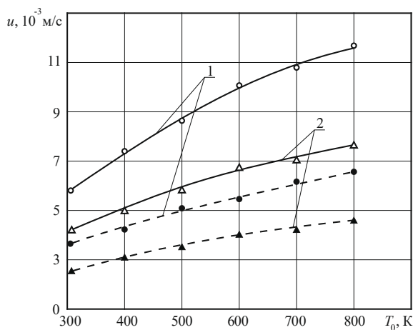
Рисунок 6. Вплив добавок парафіну на залежність швидкості горіння сумішей Al + NaNO 3 від температури нагріву ( \alpha = 1,0 , d_{ок} = 106 мкм, P = 10^5 Па): 1 – d_m = 56 мкм; 2 – d_m = 179 мкм; — суміш без добавки; - - - \varepsilon = 0,20 ; ○, ●, Δ, ▲ – експериментальні дані
