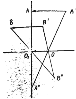
Сурет 5. O нүктесіне сәйкес T параллель көшіру мен S_0 симметриясының S_0 \circ T композициясы
