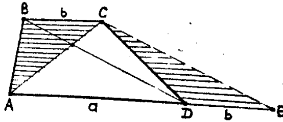
Сурет 2. \vec{g} = \vec{BC} параллель көшіруі
