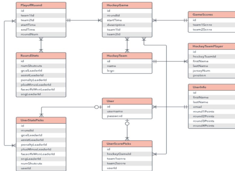
Рис. 1. Приклад ER-діаграми
