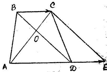
Сурет 3. AOD үшбұрыш ауданының трапеция ауданына қатынасы
