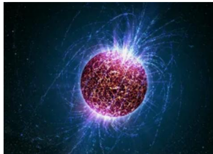
Сурет 4. Пекулярлық жұлдыз
