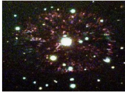
Сурет 5. Айнымалы жұлдыздар
