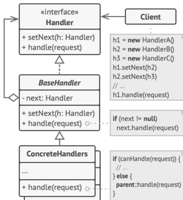
Рис. 2. Структура обробника
