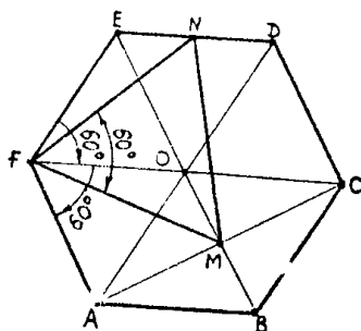
Сурет 1. MNF дұрыс үшбұрыш екенін дәлелдеу
