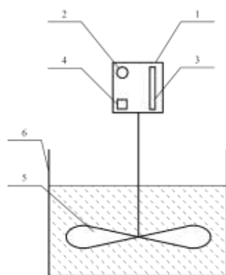
Рис. 1. Схематичне зображення електричної лопатевої мішалки: 1 – блок живлення, 2 – пристрій регулювання швидкості обертання, 3 – шкала кількості обертів, 4 – вмикач, 5 – лопаті, 6 – робоча ємність
