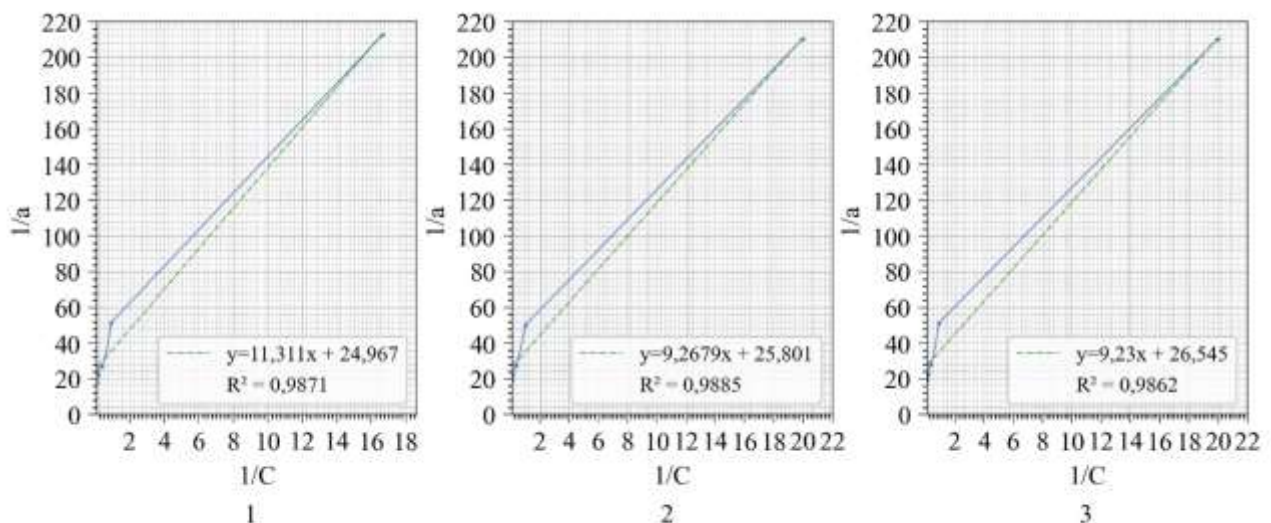
Рис. 4. Лінеаризовані ізотерми Ленгмюра адсорбції барвників: 1 – реактивного жовтого S-3R; 2 – дисперсного червоного 2C; 3 – прямого синього Direct B2RL
