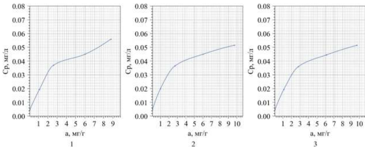
Рис. 3. Ізотерми адсорбції барвників на цеоліті: 1 – барвника реактивного жовтого S-3R; 2 – дисперсного червоного 2C; 3 – прямого синього Direct B2RL
