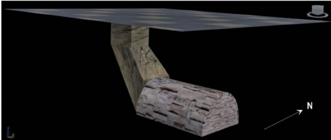
Тривимірна модель-реконструкція підземної споруди, що міститься під підлогою Іллінської церкви. Модель створена на основі георадарних досліджень 2019 р.
