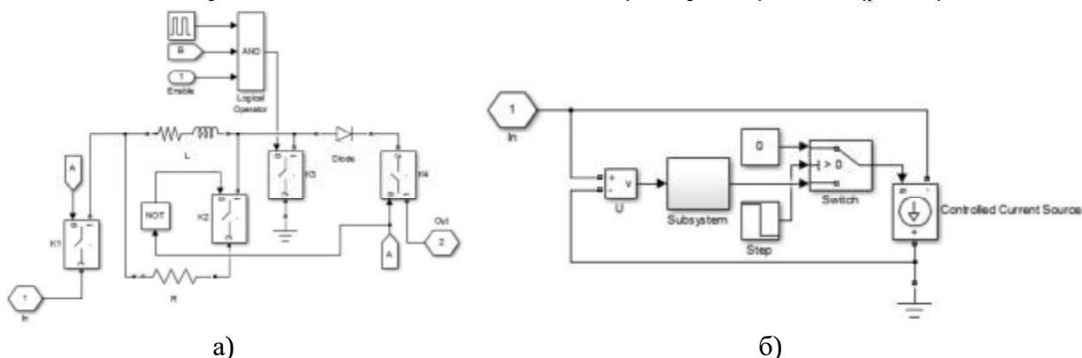
Рис. 4. Імітаційні Simulink-моделі: а) – стабілізатора напруги; б) – блоку навантаження.
