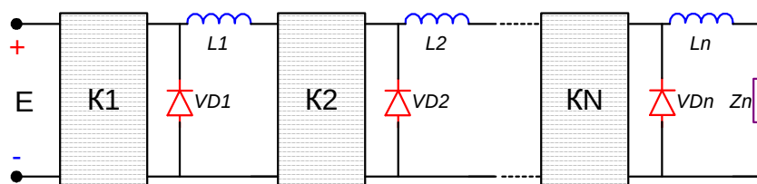
Рис. 3. Одноканальний багатокаскадний імпульсний стабілізатор напруги
