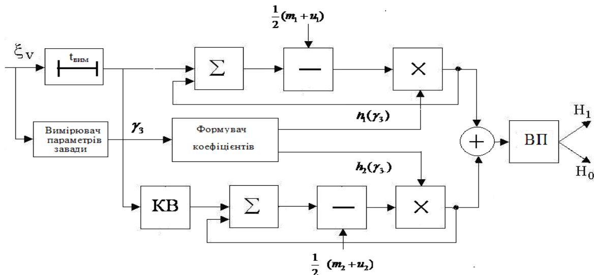
Рис. 1. Структурна схема адаптивного поліноміального виявляча при S=2
