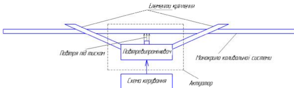
Рис. 1. Функціональна схема моделі літаючого мініробота розміром з комаху з новим типом актуатора на основі п'єзоелектричного повітрявипромінювача
