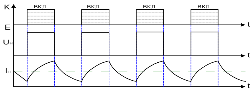
Рис. 2. Діаграма роботи однокаскадного імпульсного стабілізатора напруги
