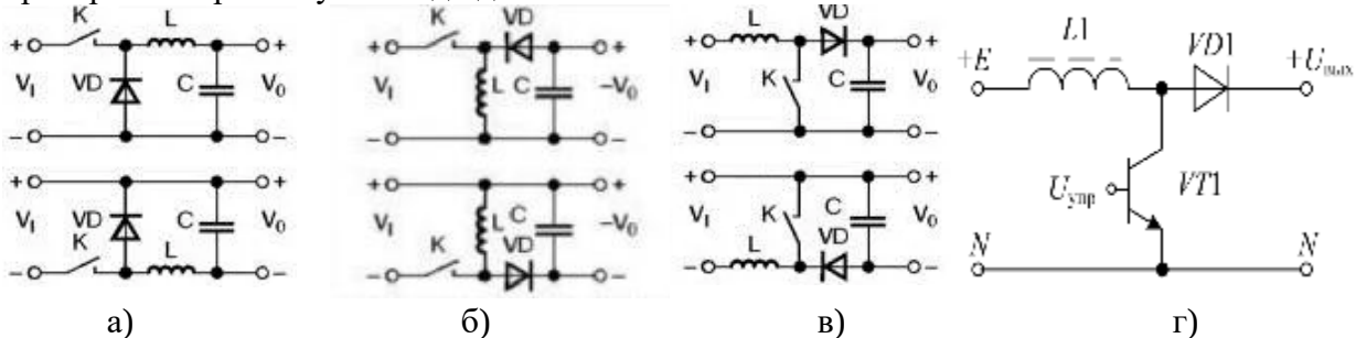
Рис. 1. Види імпульсних стабілізаторів напруги: а) – стабілізатор напруги понижуючого типу; б) – підвищуючий імпульсний стабілізатор напруги; в) – інверторний імпульсний стабілізатор напруги; г) – використання в якості ключа біполярного транзистора.
