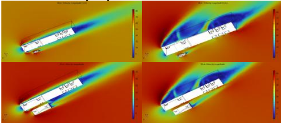
Рис. 1. Результати розрахунку обгону вантажівки мотоциклом та легковим автомобілем без врахування бокового вітру та при боковому вітрі 15 м/с
