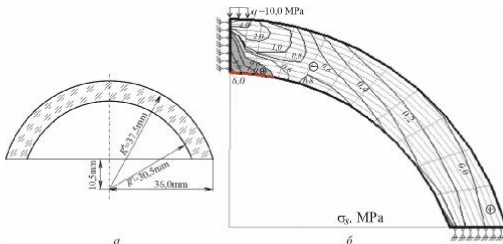
Рис. 1. Захисна оболонка – меніск: a – розрахункова схема меніска; б – області (червоні), що потребують обробки електронним променем
