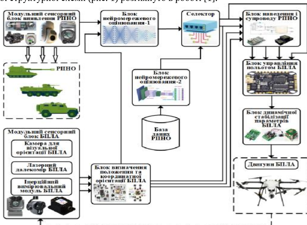
Рис. 1. Спрощена структурна схема БПЛА з реалізацією ІТ спостереження за РПНО
