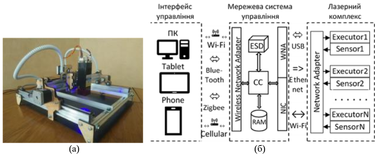
Рис. 1. Зовнішній вигляд портативного лазерного комплексу (а) та структурна схема мережевої інформаційної системи (б)
