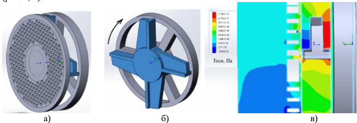
Рис. 1. 3D-модель робочої зони різального вузла вовчка та результати моделювання гідродинаміки сировини в різальному вузлі: а - комплект з приймальної решітки, ножа та вихідної решітки; б) - загальний вид ножа; в - тиск в потоці сировини, яка рухається крізь різальний вузол, Па (зображення вихідної решітки погашене)
