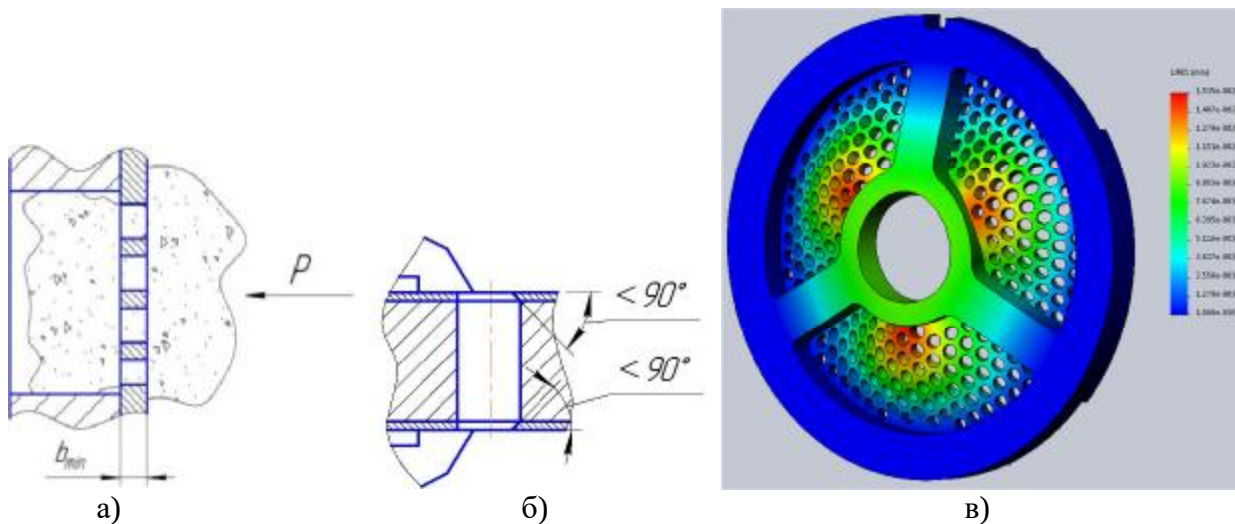
Рис. 2. Решітка вовчка вдосконаленої конструкції:
