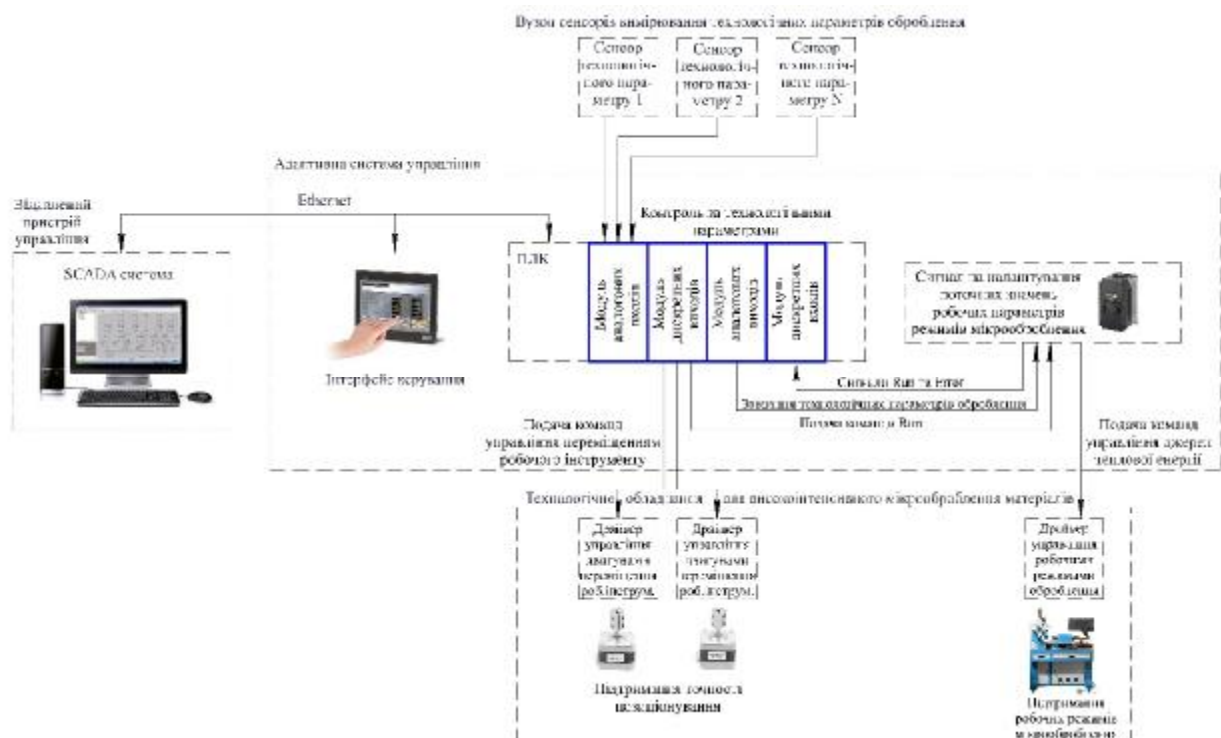
Рис. 1. Структурна схема інформаційної системи адаптивного управління процесом високоінтенсивного поверхневого мікрооброблення
