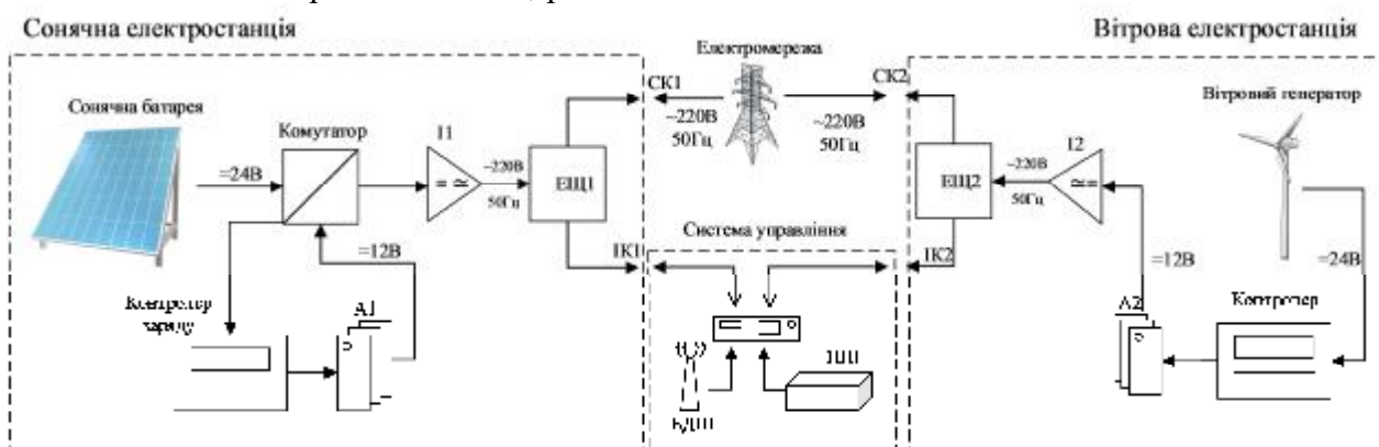
Рис.1. Функціональна схема системи управління комплексами альтернативної енергетики:
