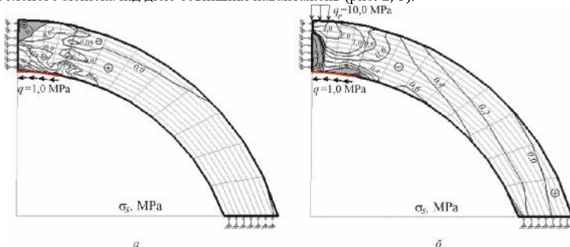
Рис. 2. Розподіл нормальних напружень: a – після обробки електронним променем; б – після обробки електронним променем під дією навантаження
