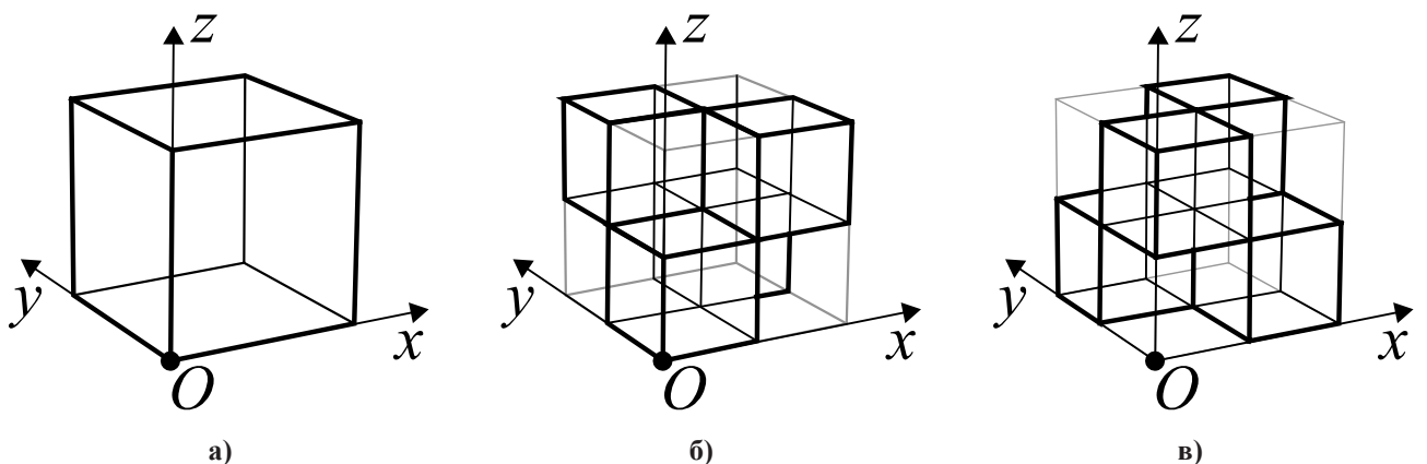
Рис 2. Куби C (а), C^+ (б) і C^- (в), що подають області визначення функцій \varphi(x, y, z) і \psi(x, y, z) у виразі (3)
