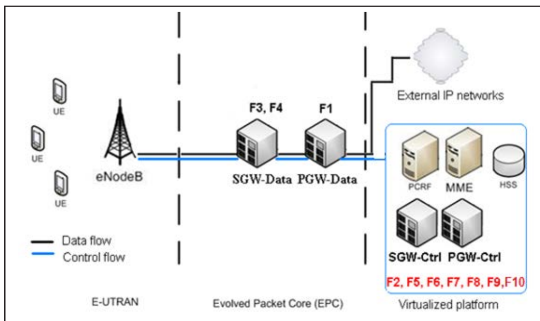
Рис. 2. Розподіл функцій ядра мережі між фізичними та віртуальними пристроями
