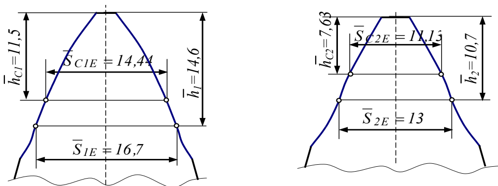
Рис. 4. Профілі зубців шестерні (а) і колеса (б) ТЗП електропоїзду ЕР2 з граничними зносами профілів за постійними хордами
