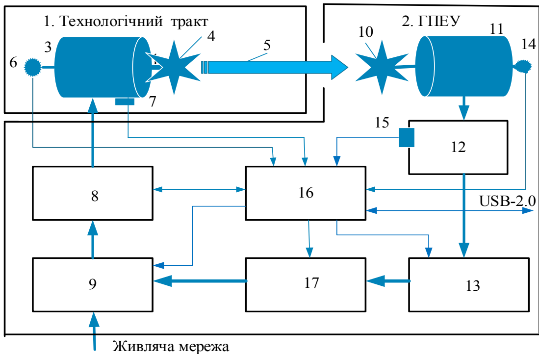
Рис.1. Блок-схема технологічний тракт і ГПЕУ
