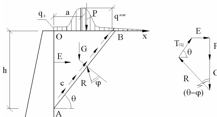
Рис. 2. Расчетная схема подпорной стенки
