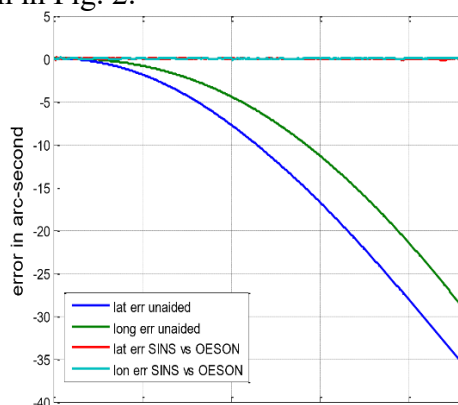
Fig. 2. Latitude and longitude errors (blue/green – uncorrected, red/turquoise – corrected)
